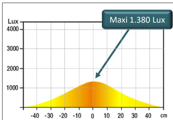
Lichtverteilung Seitenansicht bei 110 cm Abstand nach unten
