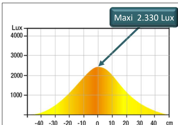
Lichtverteilung Seitenansicht bei 55 cm Abstand nach oben
