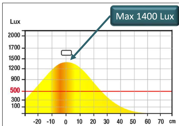
Lichtverteilung Seitenansicht bei 35 cm Abstand
